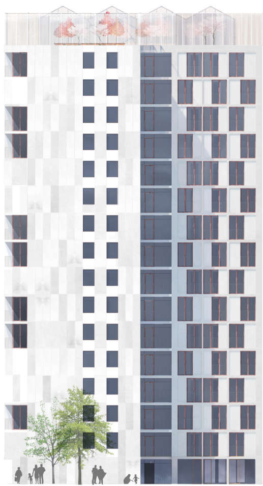
Facade Øst 1:200
