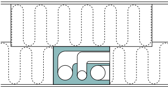
Snitprinsip vandføringer i tagetagens gulv
