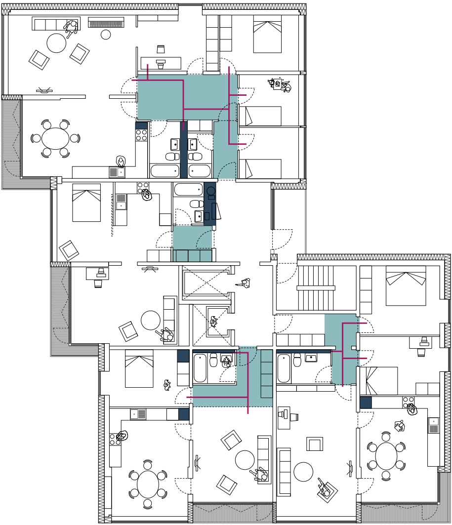
Fremtidig lejlighedsplan 1:200
