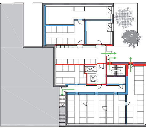
Ulsøparken 6, Lobby, Kælderetage, parkeringsniveau 1:500
