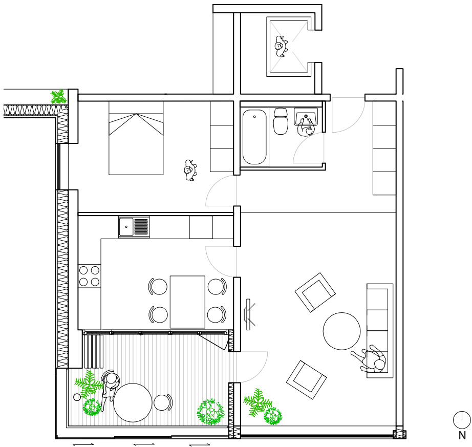
Eksempel på Lejlighedstype 2 _ Vinterhave udenfor køkken. Foldedør adskiller køkken og vinterhave. Vinterhaven har skydevinduer fra brystningshøjde og op.
