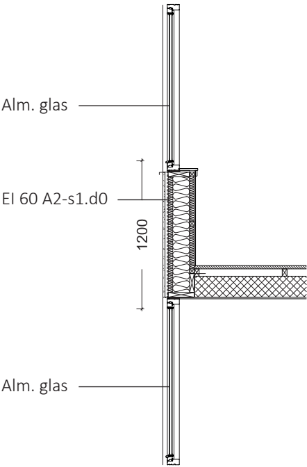
Snit A-A 1:50
