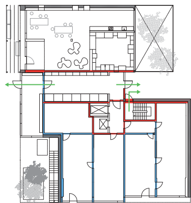
Ulsøparken 6, Lobby, Parterreetage, Strædeniveau 1:500
