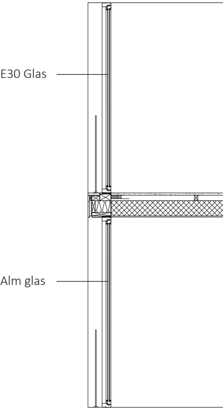
Snit B-B 1:50
