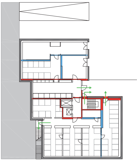
Ulsøparken 2, Lobby, Kælderetage, parkeringsniveau 1:500
